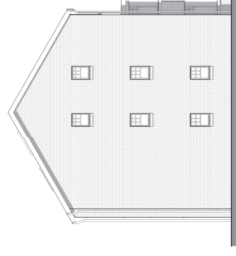
7 End Elevation - Flats 1 : 100
