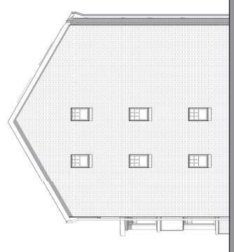
5 Side Elevations - Flats 1 : 100
